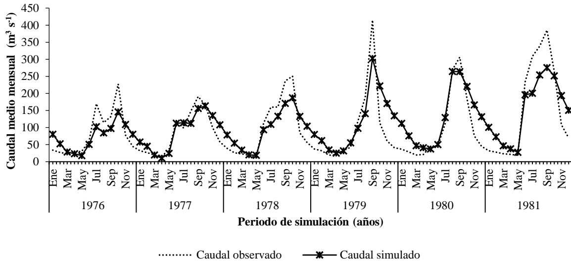
Figura 4. Caudal medio mensual, simulado por SWAT y observado de la cuenca del río Sordo, en Oaxaca, México.
