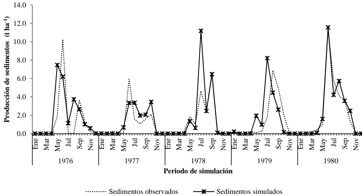
Figura 6. Producción de sedimentos simulados y observados, a nivel mensual, en la cuenca del río Sordo en Oaxaca, México.
