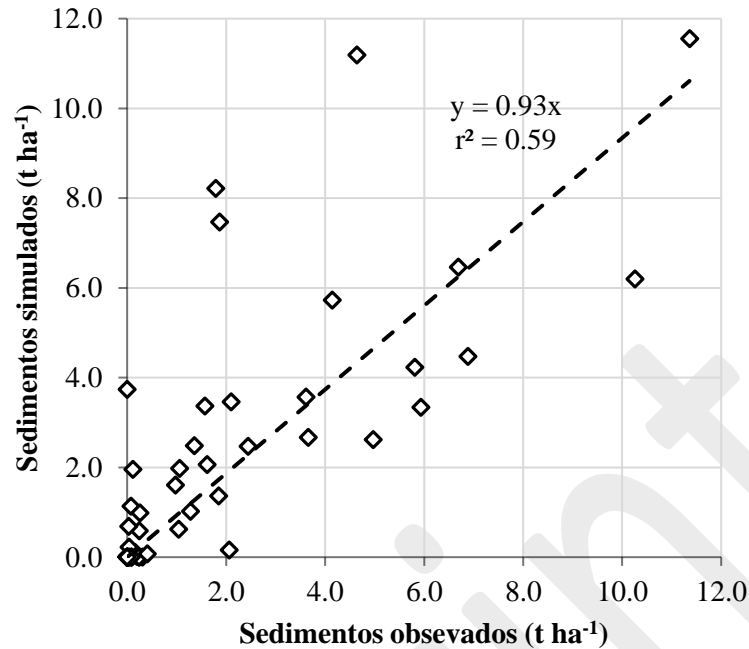
Figura 7. Comparación entre sedimentos observados y simulados por el modelo SWAT a nivel mensual, cuenca del río Sordo, Oaxaca, México.
