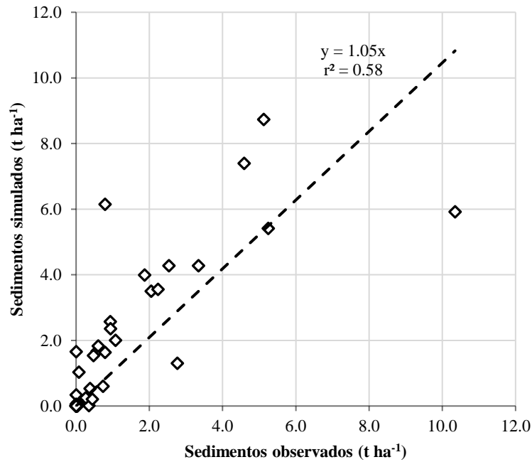
Figura 11. Comparación entre los sedimentos observados y los simulados por el modelo SWAT, a nivel mensual, durante el periodo de validación en la cuenca del río Sordo en Oaxaca, México.
