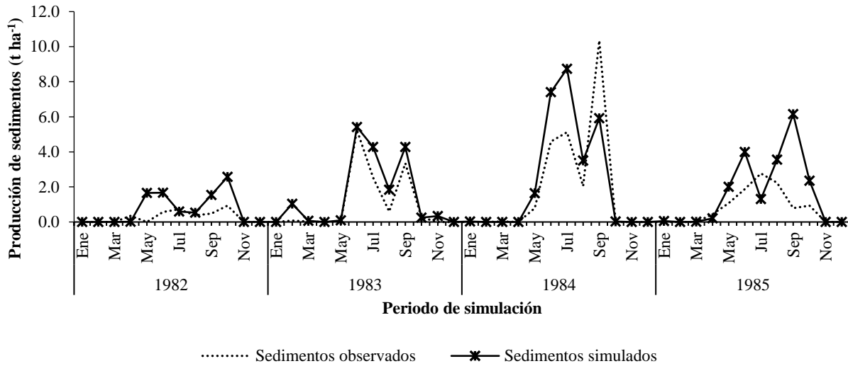
Figura 10. Producción de sedimentos simulados y observados a nivel mensual durante la etapa de validación, en la cuenca del río Sordo en Oaxaca, México.
