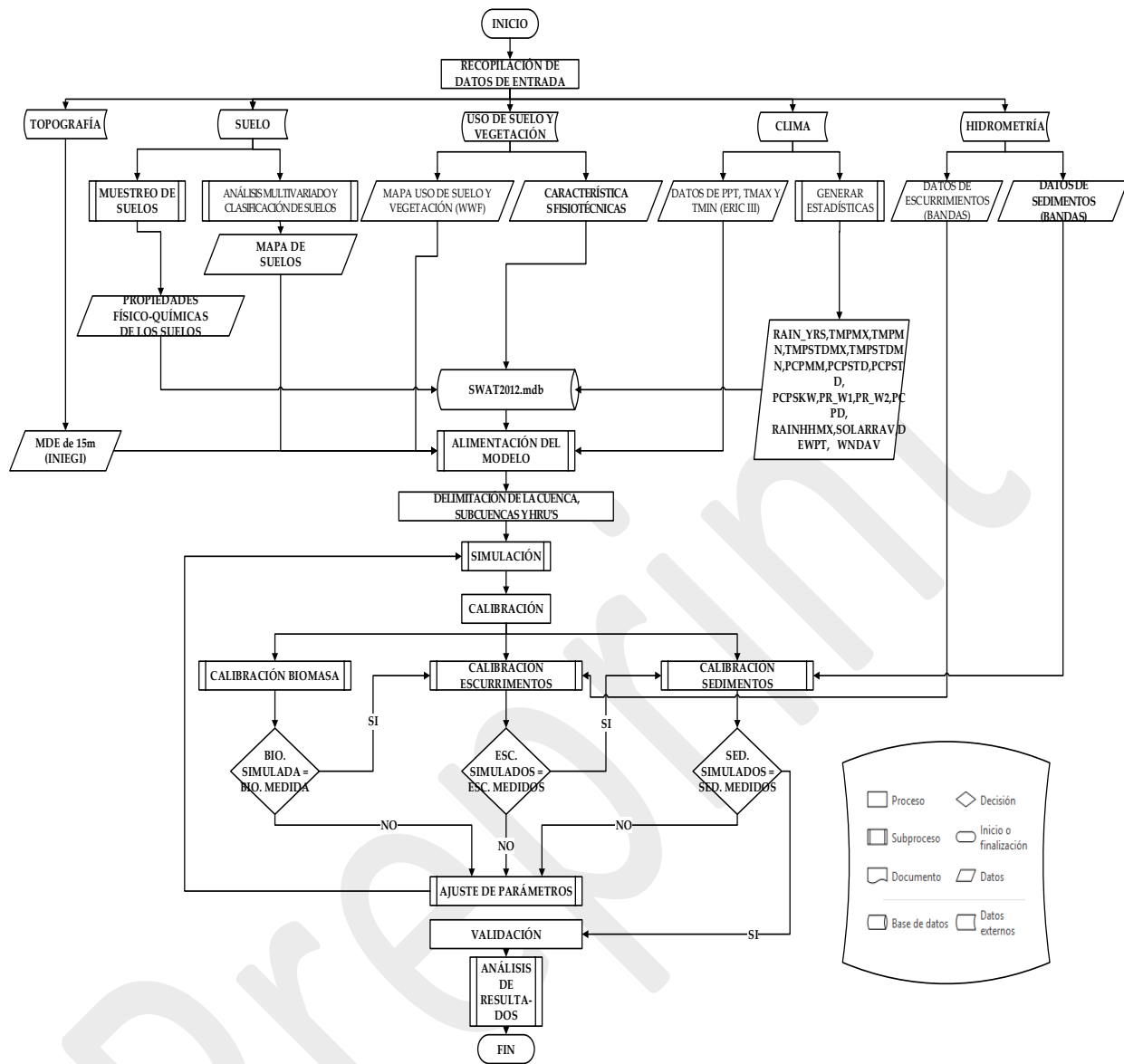
Figura 2. Diagrama de flujo de la metodología para calibrar y validar el modelo SWAT en la cuenca del río Sordo en Oaxaca, México.
