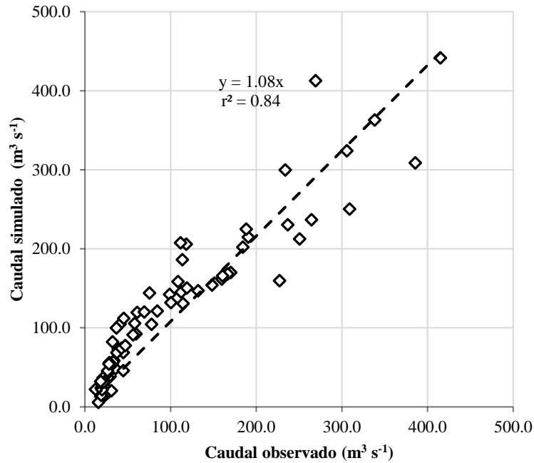
Figura 5. Comparación entre caudales medios mensuales, observados y simulados por el modelo SWAT en la cuenca del río Sordo en Oaxaca, México.
