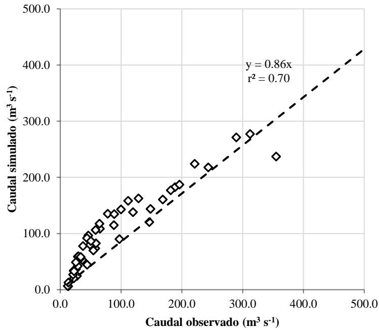
Figura 9. Comparación entre caudales observados y simulados por el modelo SWAT, a nivel mensual, durante el periodo de validación, en la cuenca del río Sordo en Oaxaca, México.
