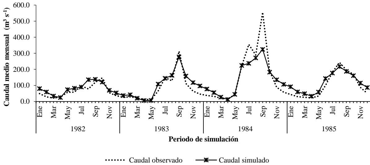
Figura 8. Caudal medio mensual simulado y observado durante la etapa de validación, de la cuenca del río Sordo en Oaxaca, México.
