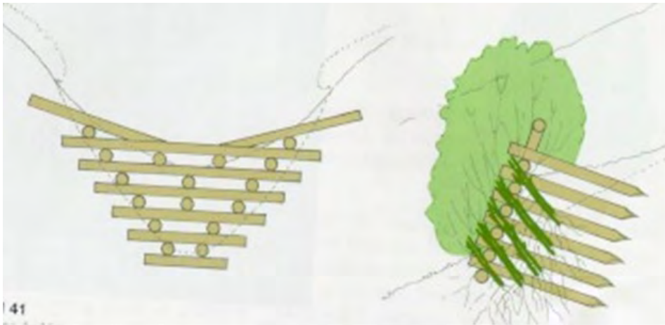
Figura 3.5.3. Colocación de represas filtrantes con estacas reñonable fuente: schiechl y stern, 2001, abb. 41
